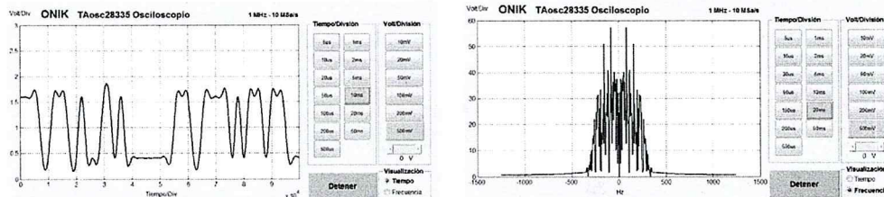
Figura: Interfaz del osciloscopio mostrando una señal en el tiempo (izquierda) e interfaz mostrando la misma señal en el dominio de la frecuencia (derecha)
