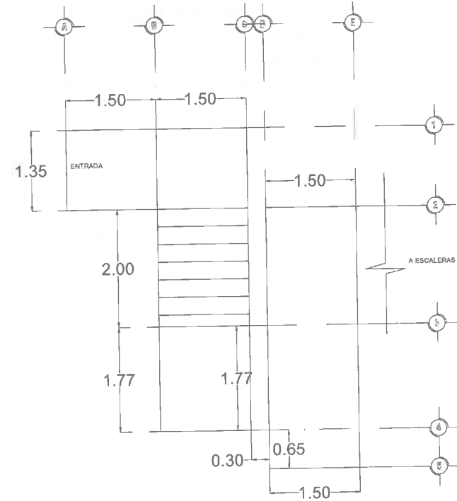
Planta Arquitectónica Baranda AREA1 ESC: 1/6
